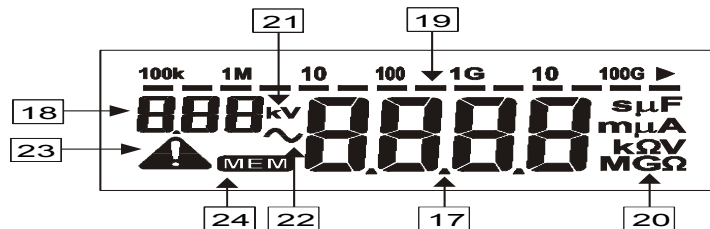
Рис.2. Жидкокристаллический дисплей
